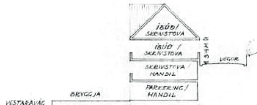
D1, VEGLEIÐANDI BYGGISKURÐUR
