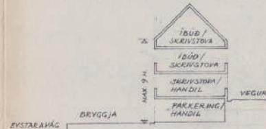
D2, SKURÐUR 1:200
